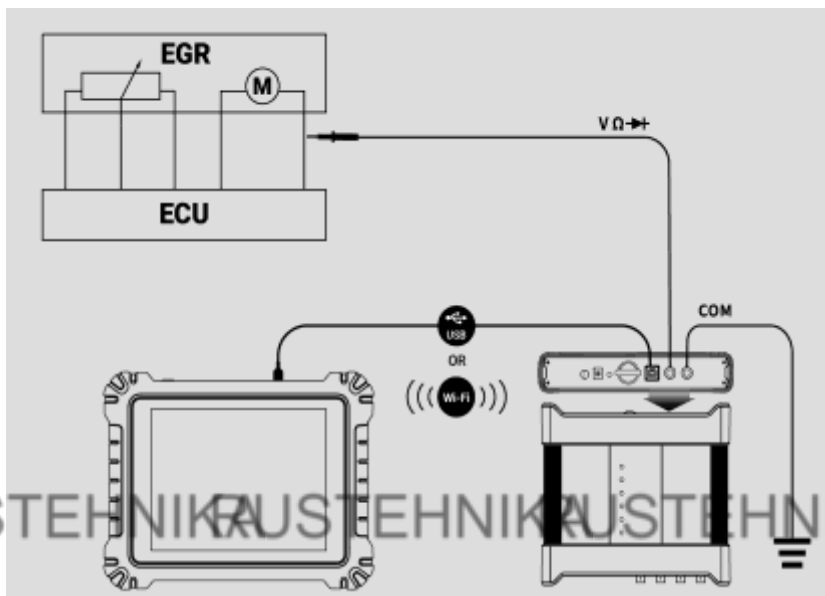
Рисунок 7-12. Пример схемы подключения к приводу исполнительного механизма
