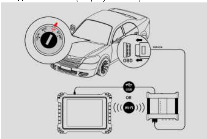
Рисунок 7-60. Пример схемы подключения к диагностическому разъёму
