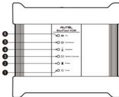
Устройство VCM1 (вид спереди)
