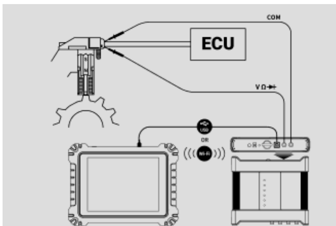
Рисунок 7-14. Пример схемы подключения при использовании прямоугольного сигнала (X+Y)
