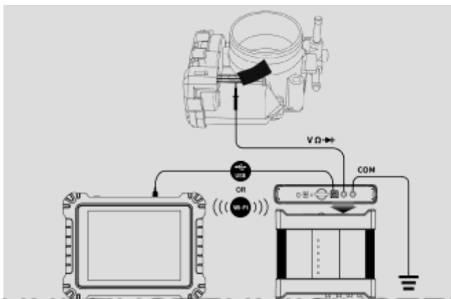
Рисунок 7-1. Пример схемы соединений
