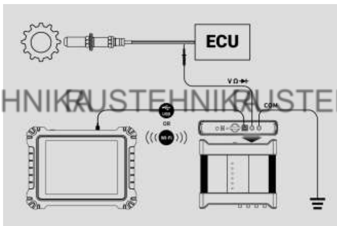
Рисунок 7-13. Пример схемы подключения при использовании прямоугольного сигнала
