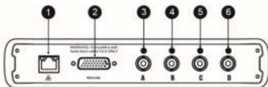
Устройство VCM1 (вид снизу)
