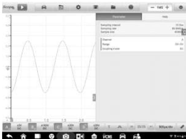
Рисунок 7-44. Пример окна параметров
