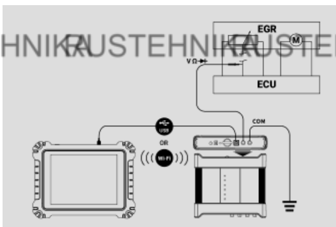
Рисунок 7-11. Пример схемы подключения для измерения постоянного напряжения
