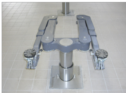
2.35 TTL с двухшарнирными захватами MINI-MAX, грузоподъемность 3,5 т
