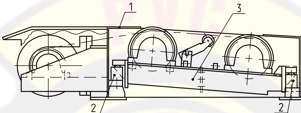
Рисунок 2 – Устройство опорное (на двух листах), лист 1
