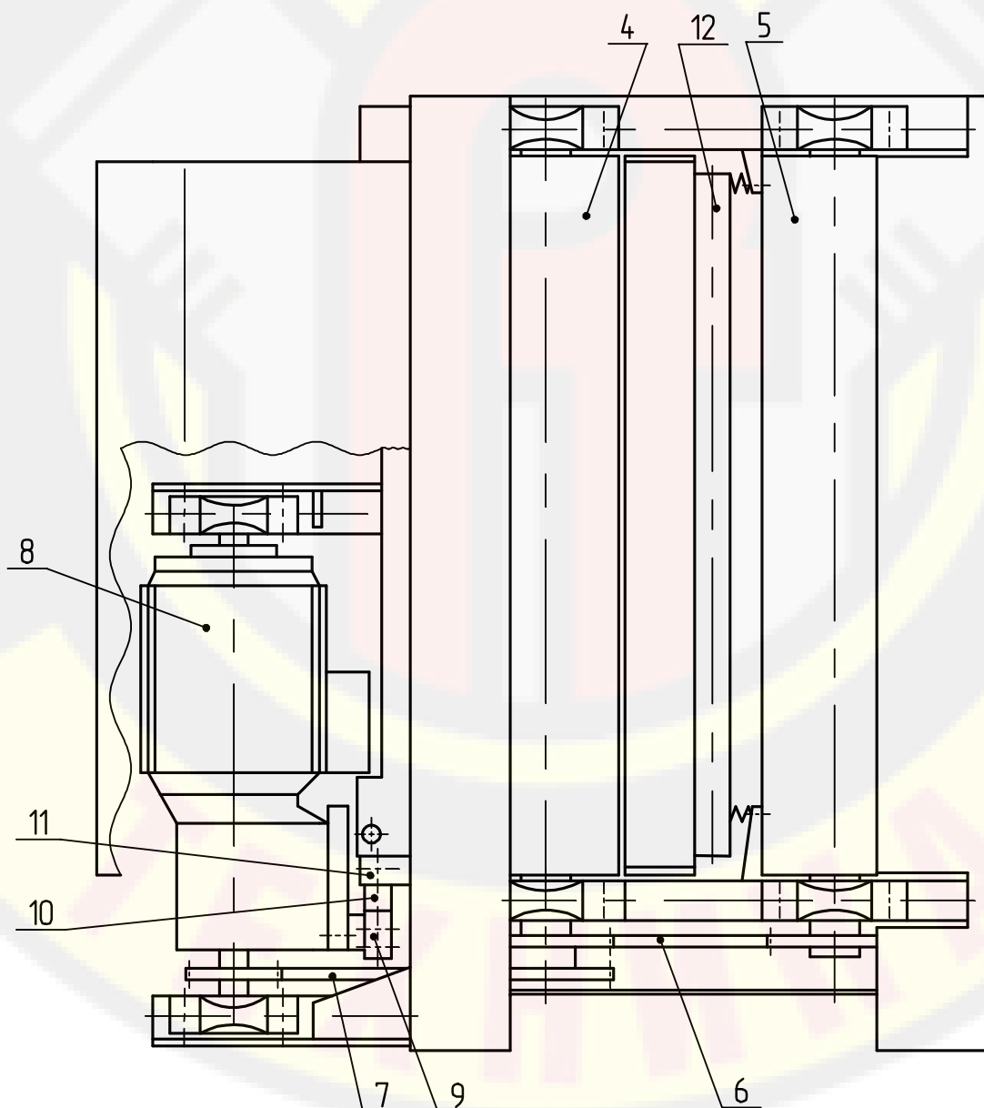
Рисунок 3 – Устройство опорное (на двух листах), лист 2
