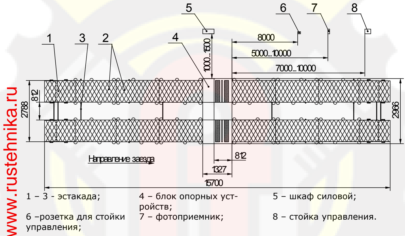
Рисунок 1 – Схема расположения основных частей стенда
