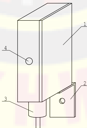
Рисунок 7 – Фотоприемник
