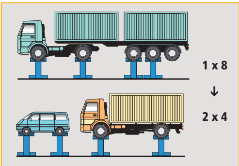
Модульная электрическая система позволяет формировать различные конфигурации (переход от 4 к 6 колоннам или 8-ми, или создание двух модулей по 4 колонны, разделив блок из 8).
