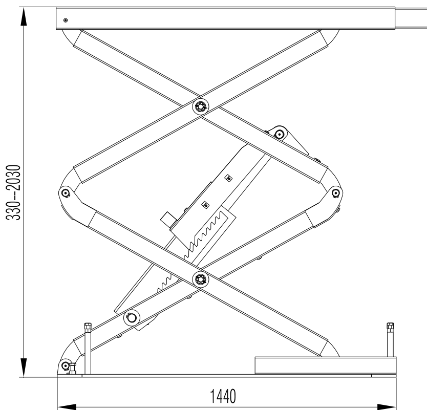
Рис. 2 - Габаритные размеры
