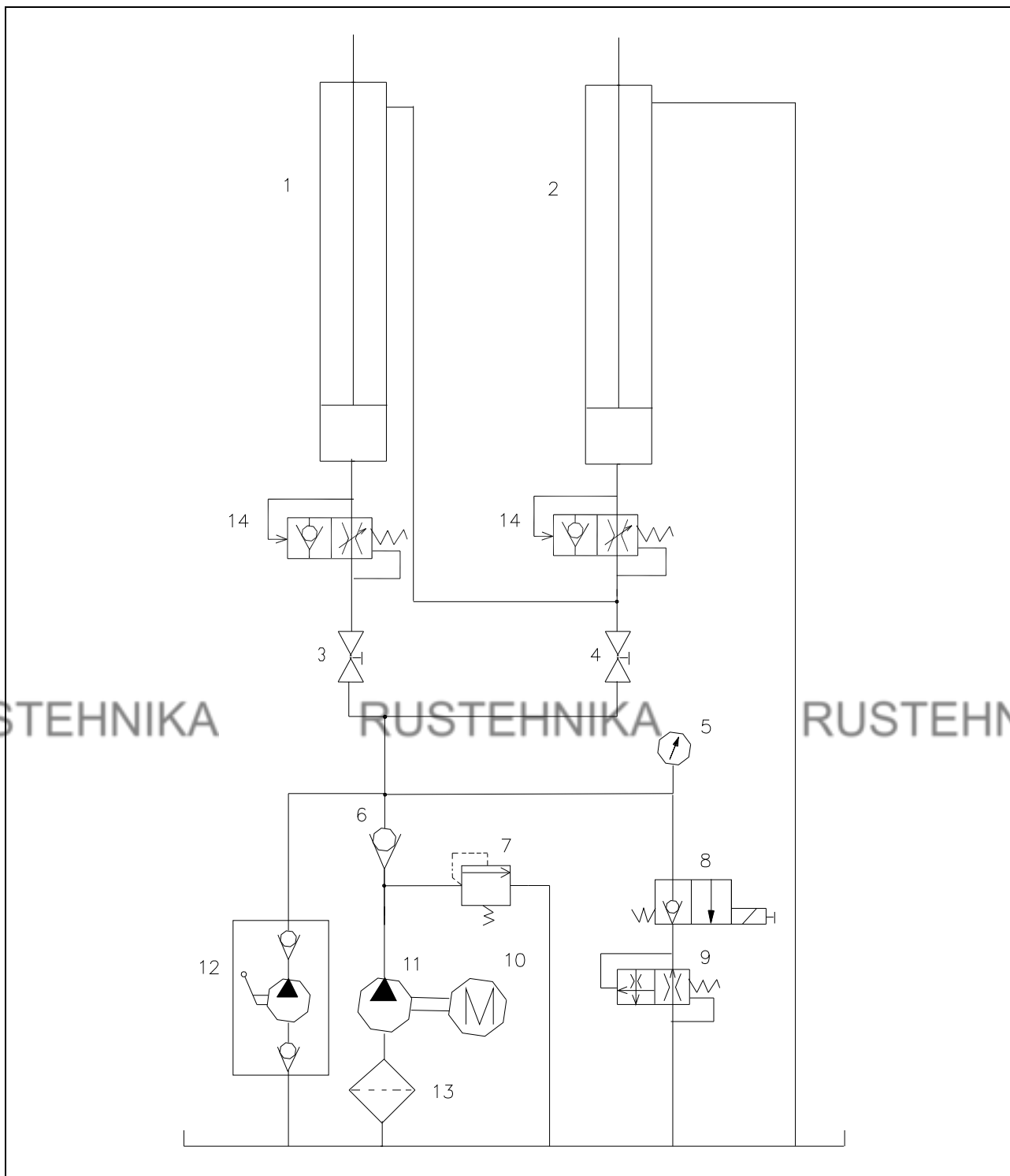
Рис. 4 – Гидросистема
