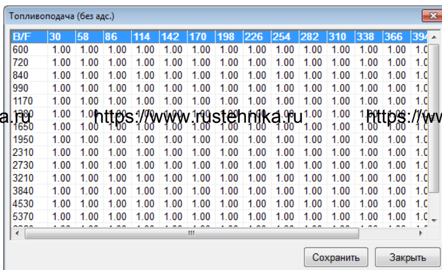
Таблицы топливоподачи
