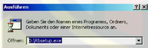
Рис.3. Ввод Rbsetup.exe
