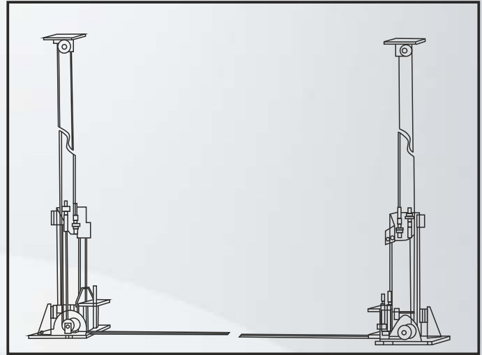
Рис.3 Установка тросов синхронизации
