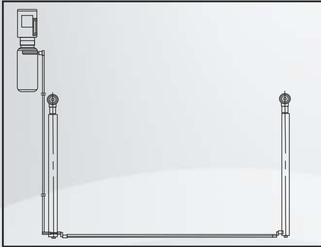
Рис. 2 Гидравлическое соединение
