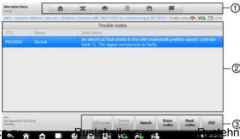
Рисунок 4-10. Пример окна считывания кодов
