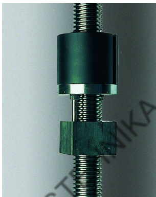
Долговечная ходовая гайка из нилатрона, гарантия 5 лет
