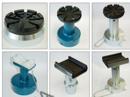
Различные адаптеры для безопасного подъема коммерческого транспорта и внедорожников
