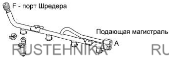
ТОПЛИВНАЯ РАМПА ВАЗ-1118 "КАЛИНА"
