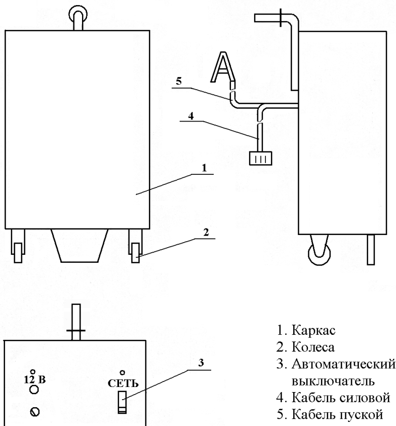
Рис. 1 Общий вид установки для запуска автомобильных двигателей
