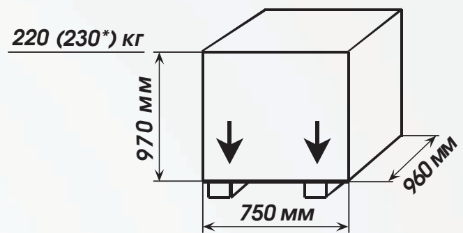
Рисунок 3 Габаритные размеры
