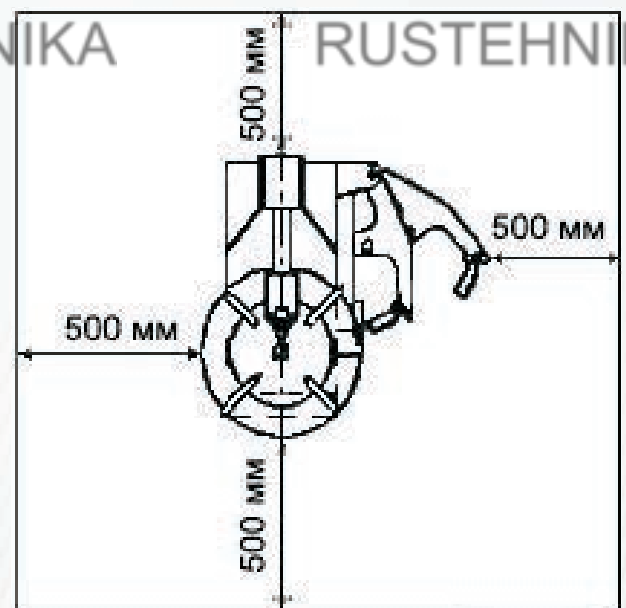
Рисунок 4.1 Установка стэнда
