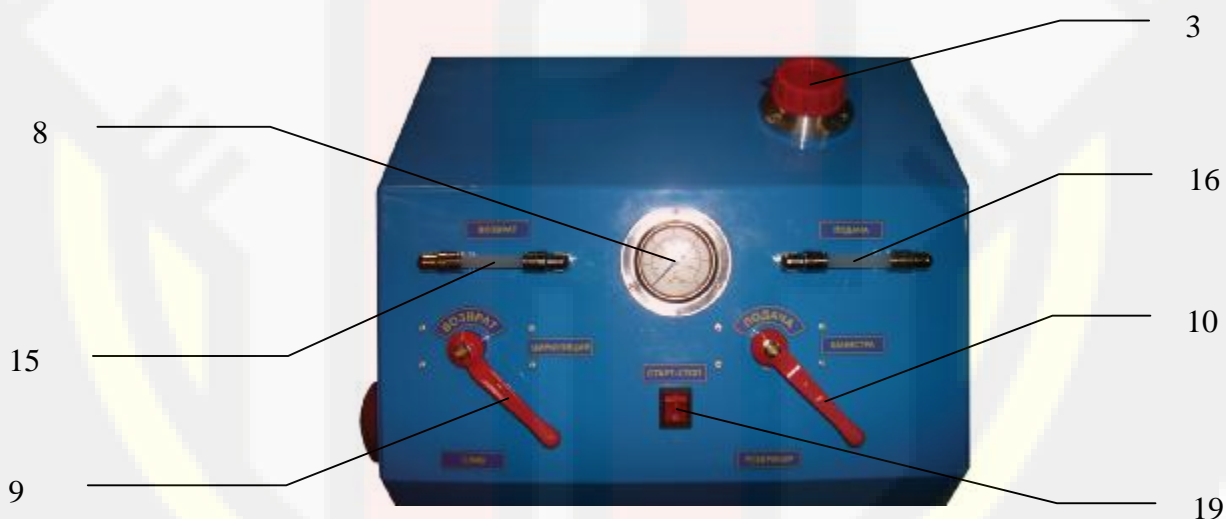
Рис.5 (панель управления)
