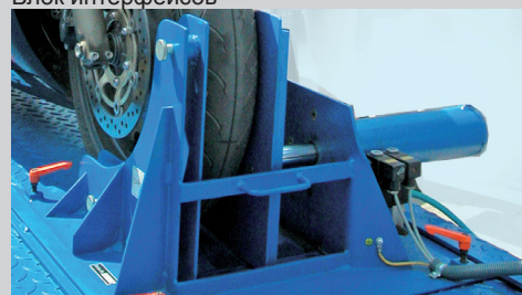
Пневматическое зажимное устройство для мотоциклов (Опция)
