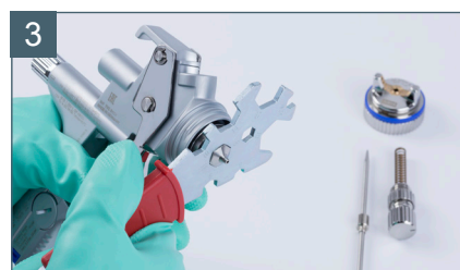
3 В завершение с помощью накидного гаечного ключа, встроенного в универсальный инструмент, вывинчивается красящая форсунка.
