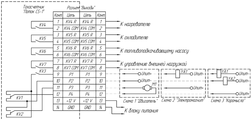
Рисунок А.5 - Схема подключения блока питания, шторы, нагревателя и охладителя тестовой жидкости, пускателя топливподкачивающего насоса и внешней нагрузки
