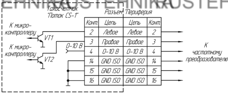
Рисунок А.3 - Схема подключения частотного преобразователя
