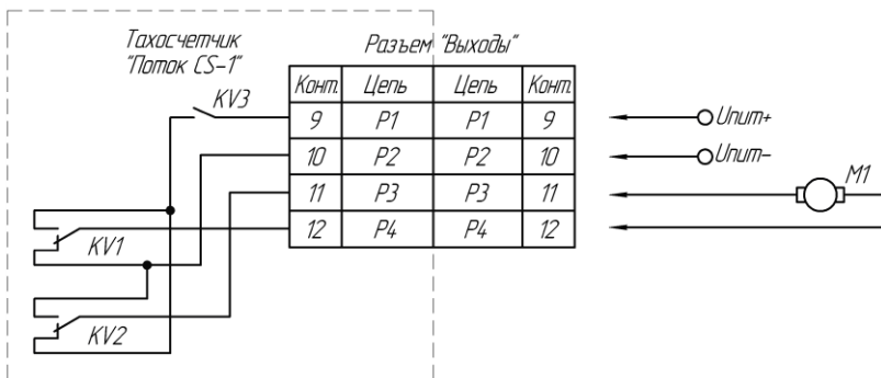
Рисунок 4.1 - Управление шторкой. Схема 1 "Двигатель"
