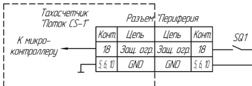
Рисунок А.7 - Схема подключения концевого выключателя защитного ограждения
