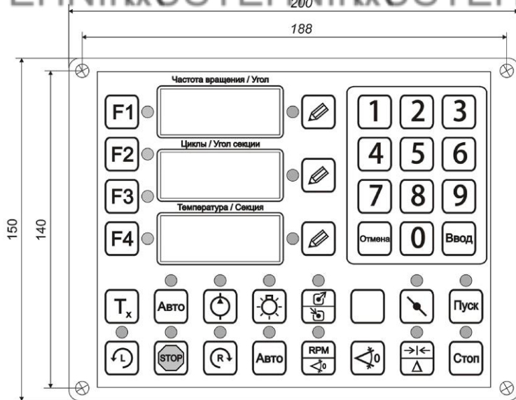
Рисунок 1.1 - Вид спереди. Исполнение 1
