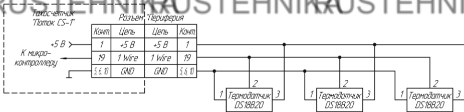
Рисунок А.6 - Схема подключения температурных датчиков
