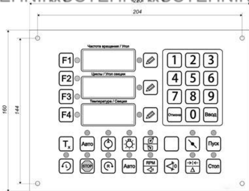
Рисунок 1.3 — Передняя панель устройства. Исполнение 2
