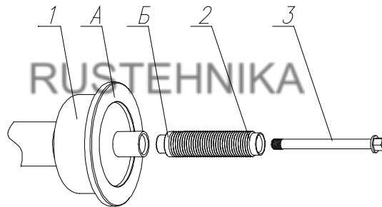
Рисунок 4.2 – Сборка вала
