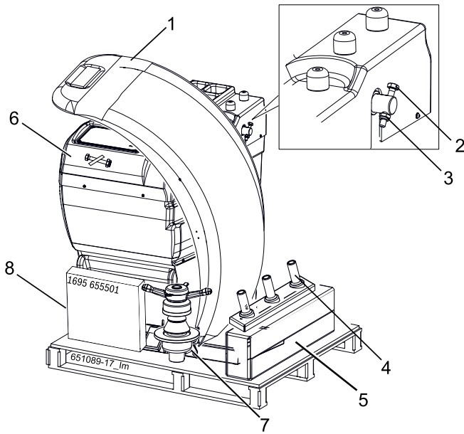
Fig. 1: Оснащение SBM 260 AW
