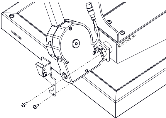
Fig. 8: Крепление пластинки концевой останова
