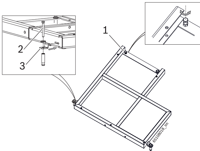
Fig. 6: Фиксация SBM 260 AW
