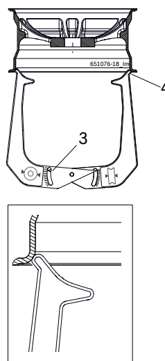
Fig. 12: Считывание данных обода с помощью измерительного циркуля
