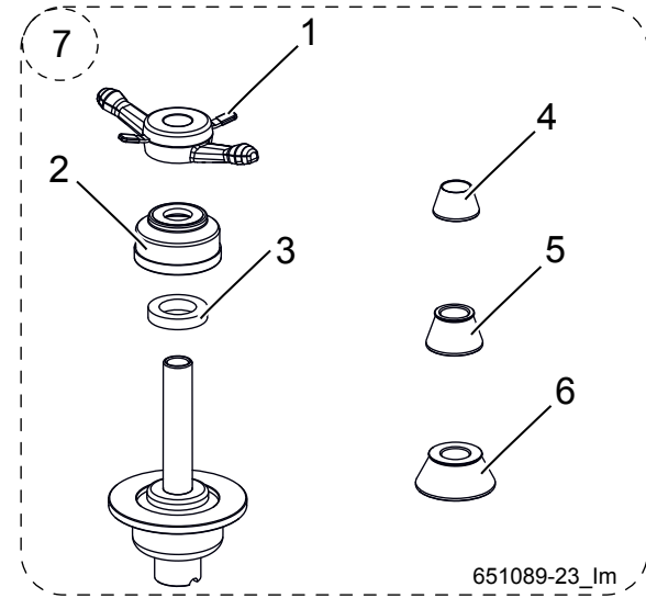
Fig. 3: Быстрое коническое соединение 1 695 602 400
