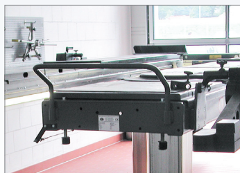
Стандартный упор U-образной формы
