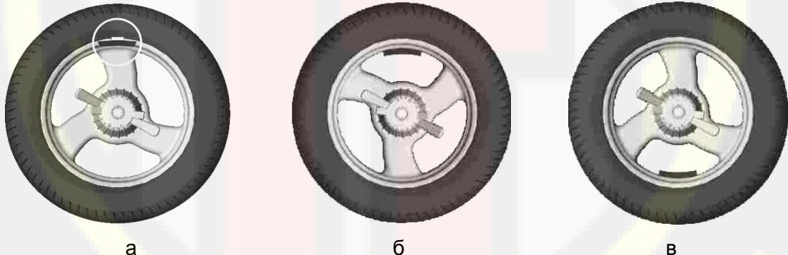
а – груз со скобой установлен в положение «12 часов» б – ленточный груз установлен в положение «12 часов» в – ленточный груз установлен в положение «6 часов»
