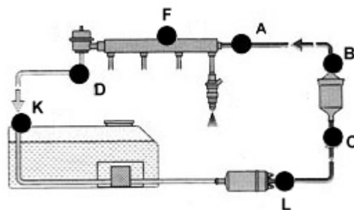
Система L- JETRONIC/ MOTRONIC с топливным электронасосом, установленном в топливопроводе последовательно с топливным баком
