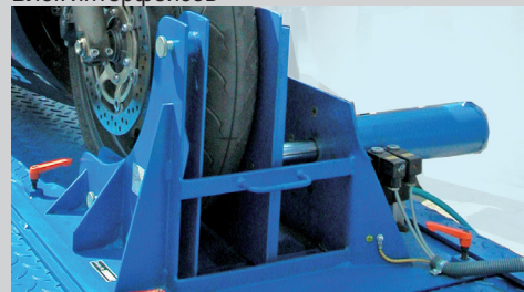
Пневматическое зажимное устройство для мотоциклов (Опция)
