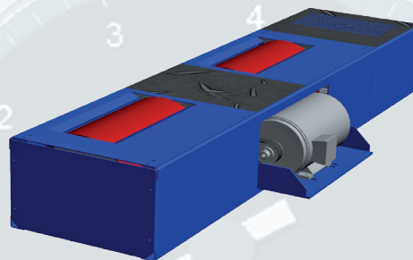
Версия стенда MSR 500 с одним роликовым агрегатом
