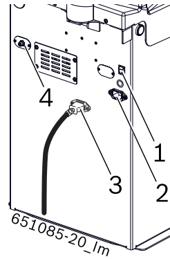
Fig. 19: Подключение к электропитанию - задняя сторона SBM 135 A
