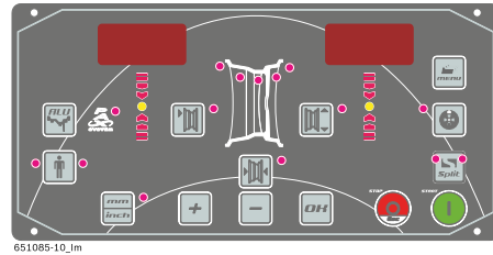
Fig. 21: Кнопки на панели управления/панели отображения
