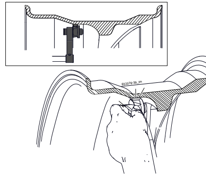
Fig. 45: Пример применения внешнего адгезивного груза
