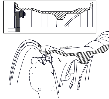
Fig. 44: Пример применения внутреннего адгезивного груза
