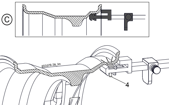
Fig. 49: Пример применения внешнего адгезивного груза
