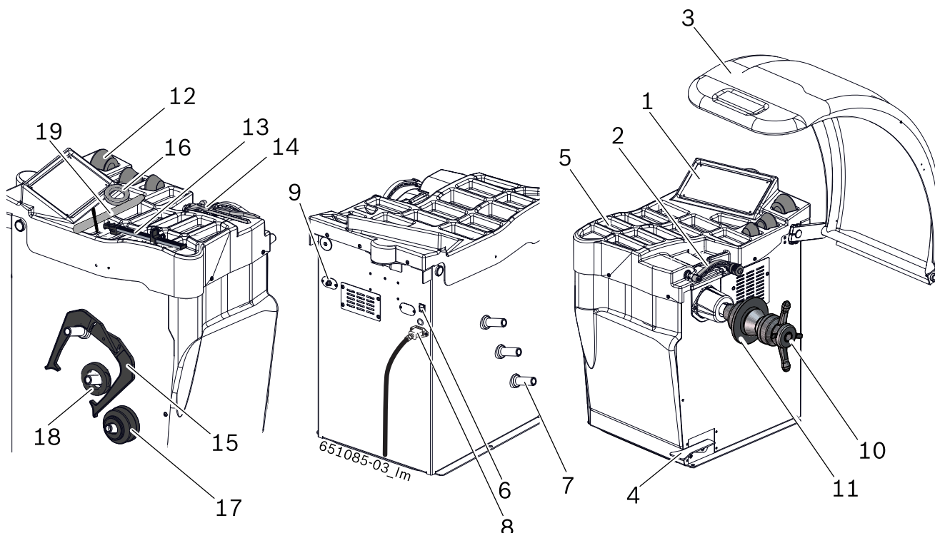
Fig. 5: SBM 135 A
