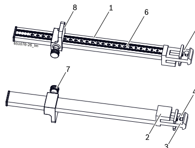
Fig. 46: Калибр позиционирования грузов
