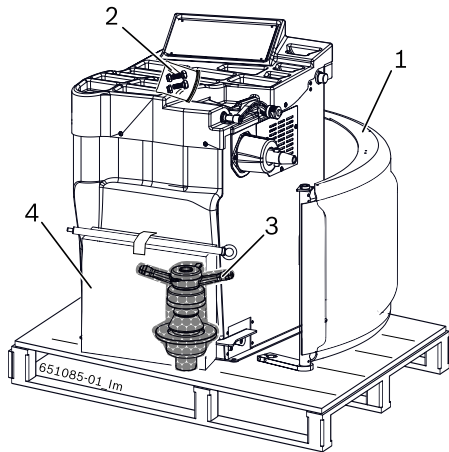
Fig. 1: Оснащение SBM 135 A
