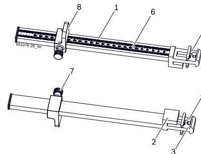
Fig. 36: Калибр позиционирования грузов
