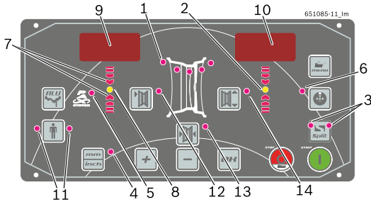
Fig. 20: Светодиоды на панели управления/панели отображения
