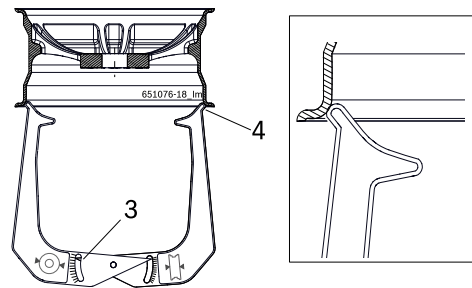
Fig. 33: Считывание данных обода с помощью измерительного циркуля
