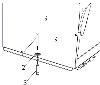
Fig. 16: Фиксация SBM 135 A
