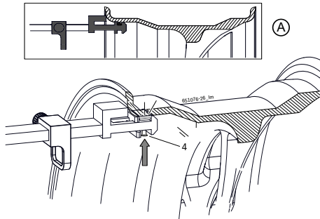
Fig. 48: Пример применения внутреннего адгезивного груза
