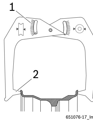
Fig. 34: Считывание данных обода с помощью измерительного циркуля
