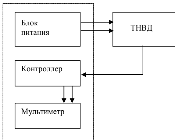
Рисунок 2. Структурная схема устройства
