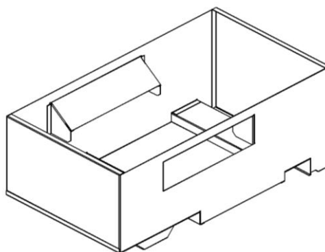
Рис.2. Перфорированный ящик для сбора гранул.
