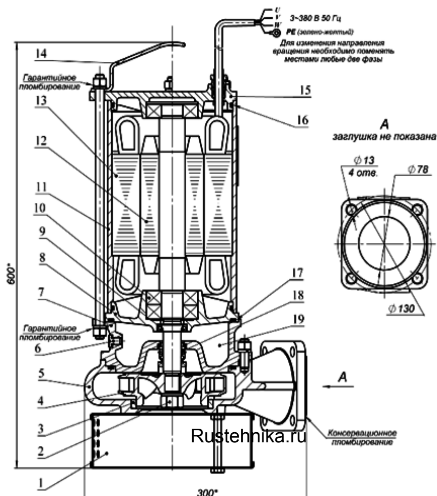
Рис.10 Устройство электронасоса
