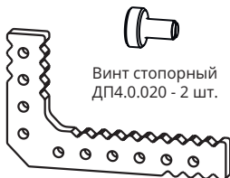
Упор ДП4-11.22.016 - 1 шт.
