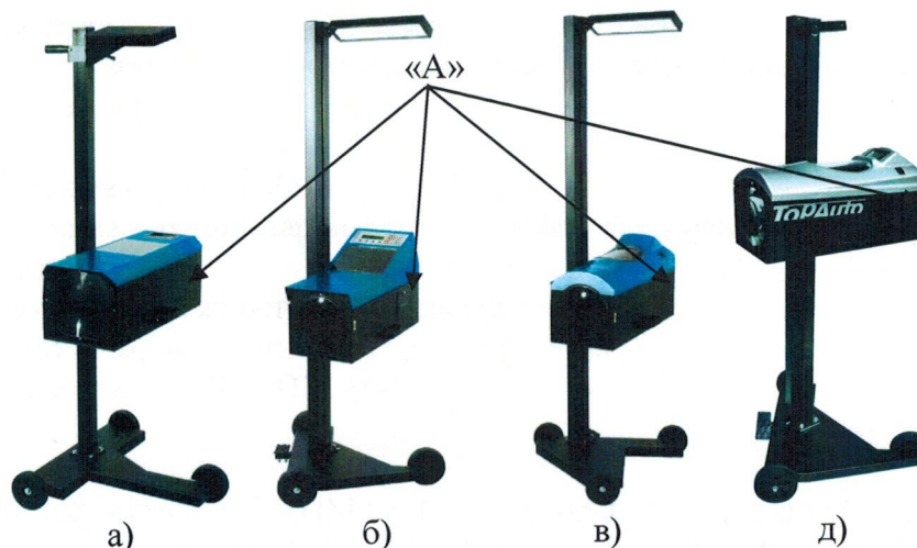
Рисунок 1 - Общий вид приборов для измерений параметров света фар автотранспортных средств, модификации НВА18К (а), НВА19К (а), НВА19D (а), НВА24К (а), НВА24UK (а), НВА25 (б), НВА26(а), НВА26D (а), НВА28 (а), НВА30 (в), НВА31PLUS (в), НВА35 (д)
