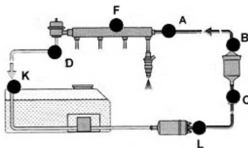
Система L- JETRONIC/ MOTRONIC с топливным электронасосом, установленным в топливопроводе последовательно с топливным баком
