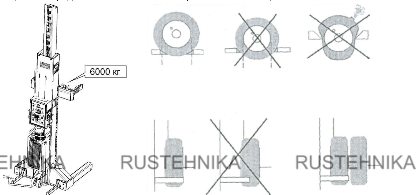
Рисунок 5.1 - Рекомендации безопасного захвата за колеса
