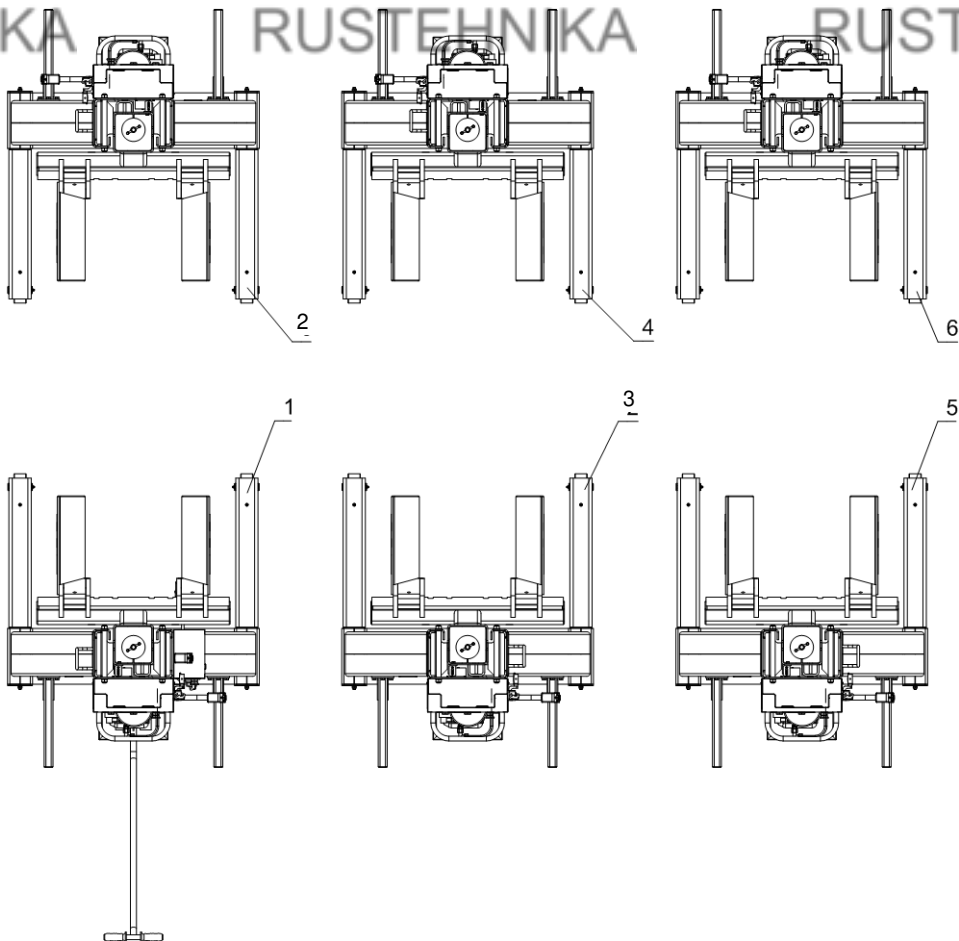
Рисунок 4.2 - Общий вид подъемника ПГП-36000/6
