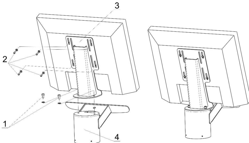
Рисунок 4.7 - Установка монитора
