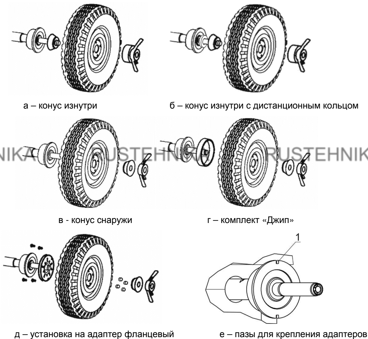
Рисунок 5.3 – Установка колеса
