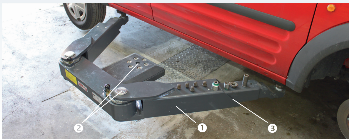
Подхват за колесо VZ 971348
