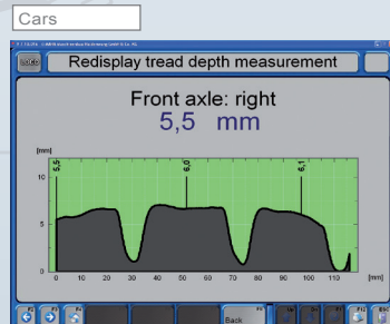
Измерение глубины протектора шины ТМ 1000 автоматически измеряет глубину протектора по всей окружности и ширине шины
