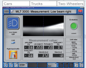
Тест фар Точное определение установки головных фар с помощью CMOS камеры
