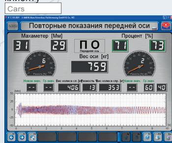
Тест амортизаторов Ясное графическое и цифровое представление измеренной информации.
