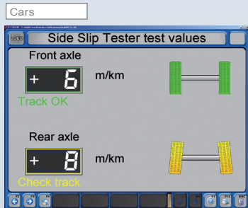
Тест бокового увода Ясное отображение результатов по осям
