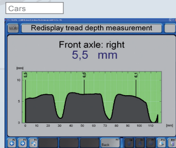
Измерение глубины протектора шины ТМ 1000 автоматически измеряет глубину протектора по всей окружности и ширине шины
