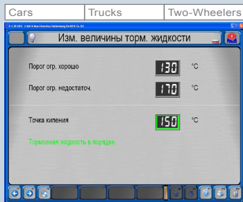
Тест тормозной жидкости Точное определение температуры кипения тормозной жидкости
