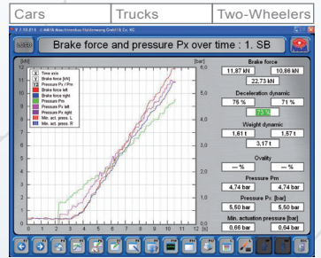
Графики Графическое представление тормозных сил во времени или в зависимости от усилия нажатия на педаль тормоза
