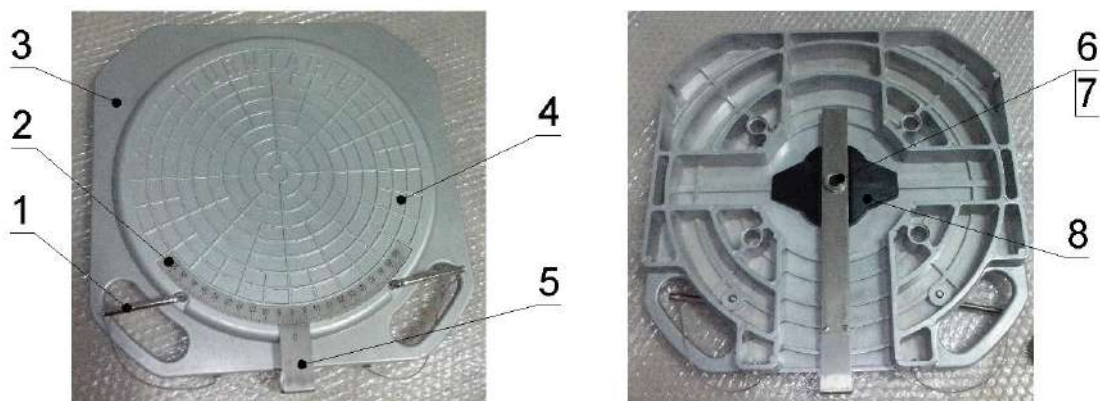
Рис. 1. Опора поворотная.
