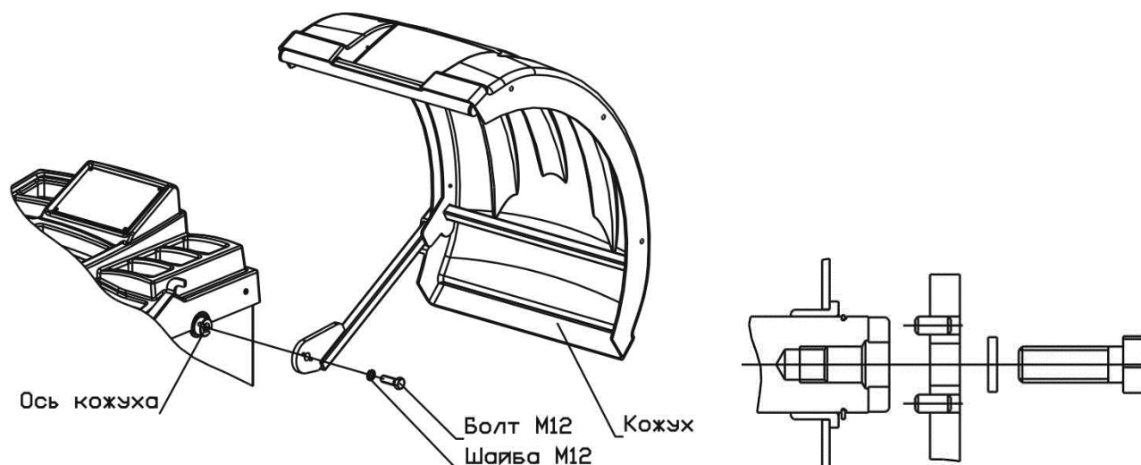
Рисунок 4.7 – Монтаж кожуха
